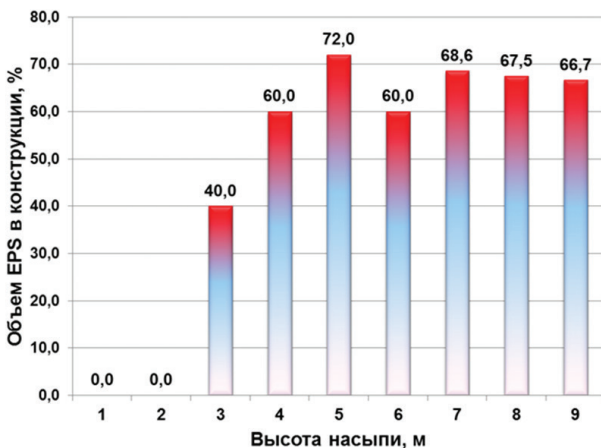
Рис. 3. Рациональный объем EPS в комбинированной насыпи, %
